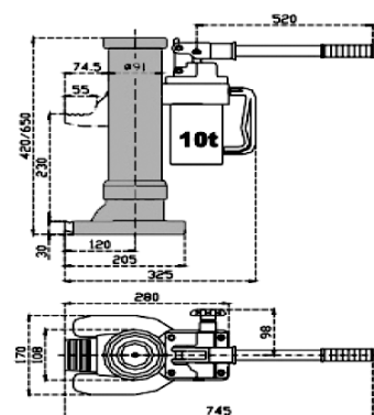
TJ-10E
