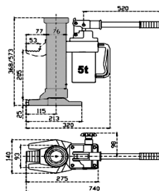
TJ-5E
